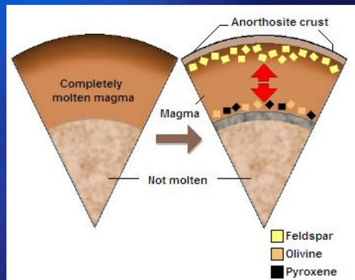
Distilarea crustei lunare
