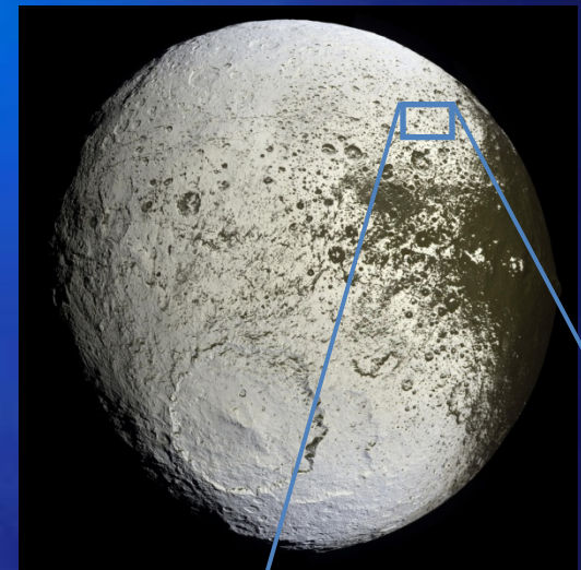
Japet, neigeux
